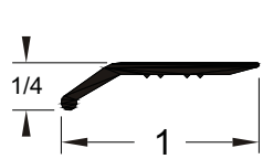
7600 A,G Binder Bar 3', 6', or 12'
